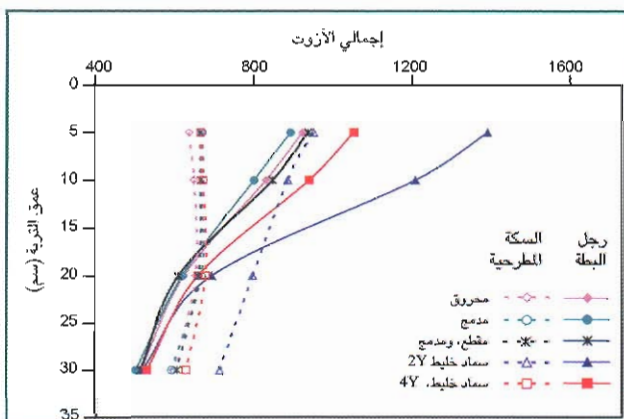
الشكل 15. إجمالي الأزوت في التربة ومعاملات إدارة التبن/السماد الخليط في تجربة لمدة سبع سنوات في تل حديا، سورية.
