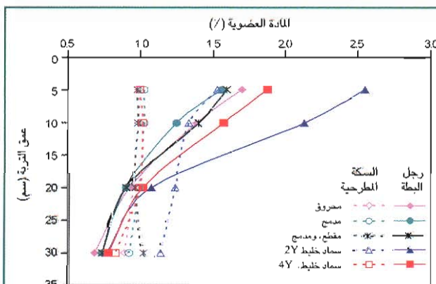
الشكل 14. تراكيز المادة العضوية في التربة في معاملات مختلفة للحراثة وإدارة التبن في تجربة لسبع سنوات في تل حديا، سورية. وقد استخدم محراث رجل البطة للحراثة السطحية في حراثة الحفظ، واستخدم محراث السكة المطرحة القلاب للحراثة العميقة في الحراثة التقليدية. وأضيف السماد الخليط كل سنتين أو أربع في معامليتين تم خلالهما إدخال بقايا المحاصيل والتبن المفروم في التربة.
