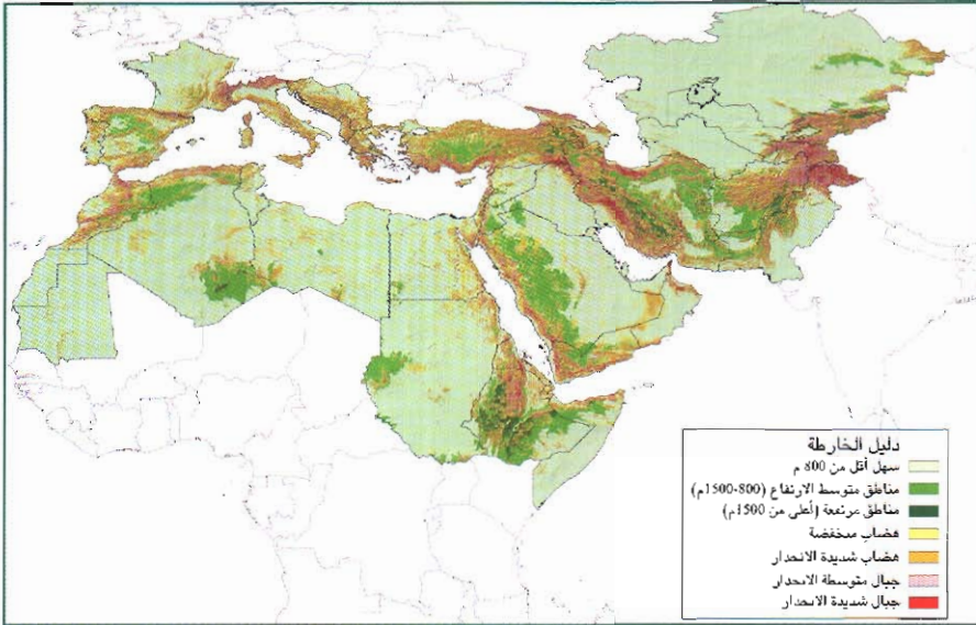
الشكل 31. خارطة جديدة لتضاريس CWANA، تعكس كثافة التضاريس (الوعورة) والارتفاعات.
